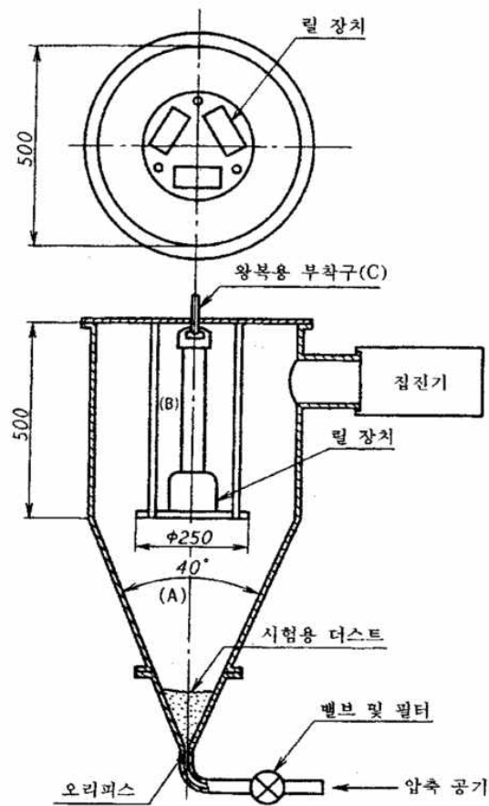
<그림 12> 방진 시험 장치
