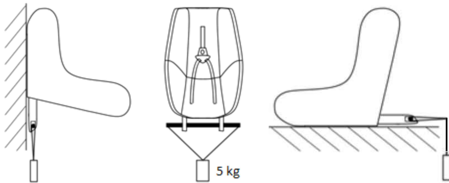
<그림 20> ISOFIX 연결부
